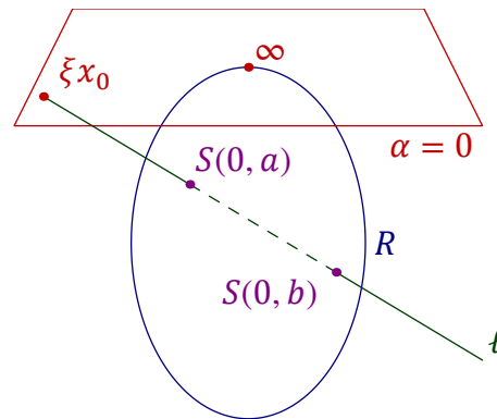
Рис. 23◊6. Пучок с двумя простыми конусами.
