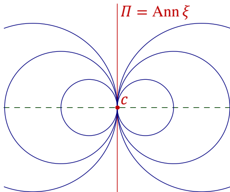
Рис. 23◊8. Пучок соприкасающихся сфер.
