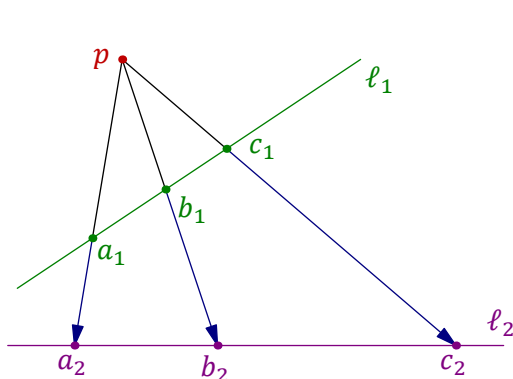
Рис. 18◊3. Перспектива p : \ell_1 \rightarrow \ell_2 .
